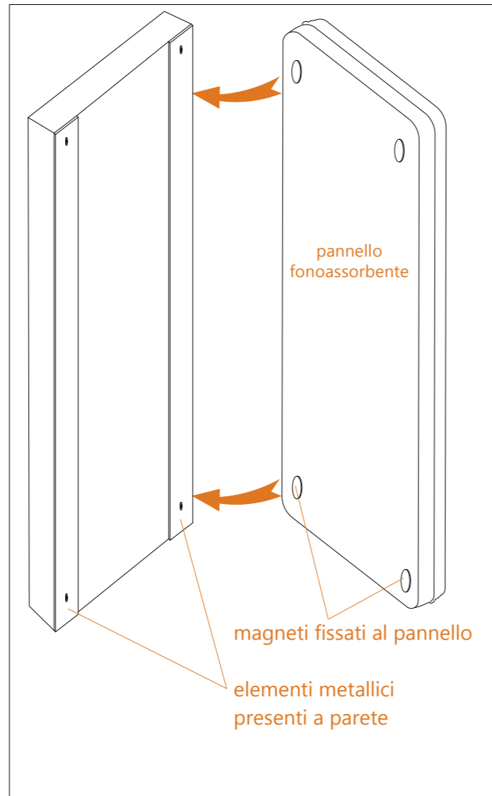
Fissaggio magnetico removibile / Magnetic fixing
